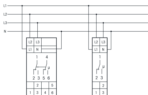
NR12-002-3x230V
