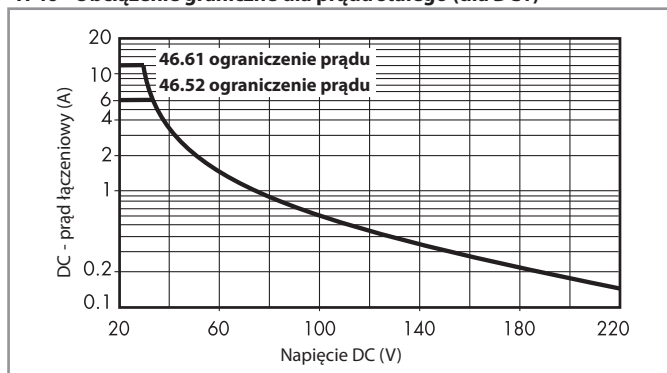
H 46 - Obciążenie graniczne dla prądu stałego (dla DC1)
