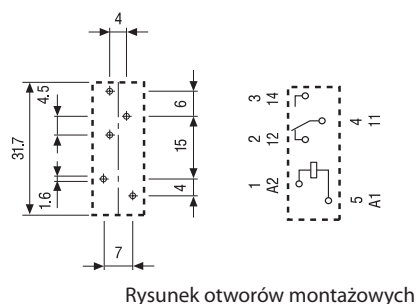
Rysunek otworów montażowych
