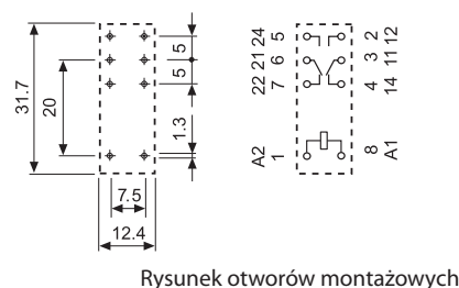
Rysunek otworów montażowych
