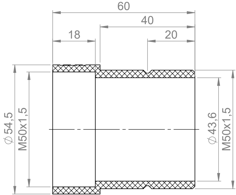
SCHNITT A-A
