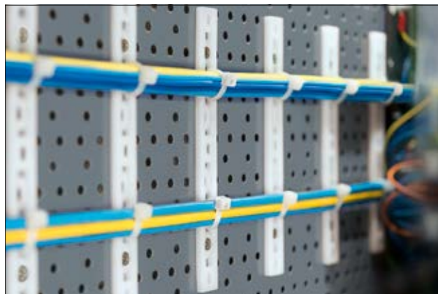
Listwy mocujące MP, przykręcane.
